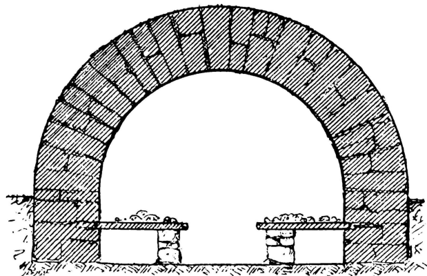
Sezione
